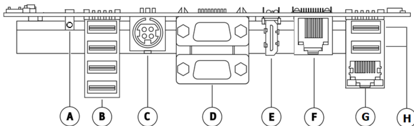
Рисунок 4. Интерфейсы:
