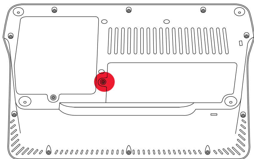
Рисунок 5. Расположение винта крепления крышки интерфейсных портов
