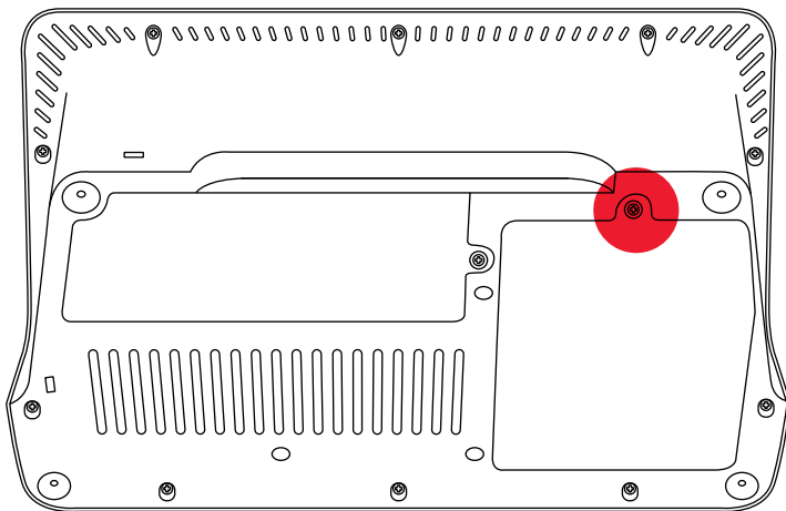
Рисунок 16. Установка и закрепление крышки
