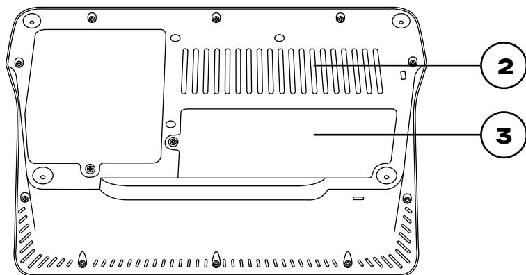
Рисунок 2. Вид снизу
