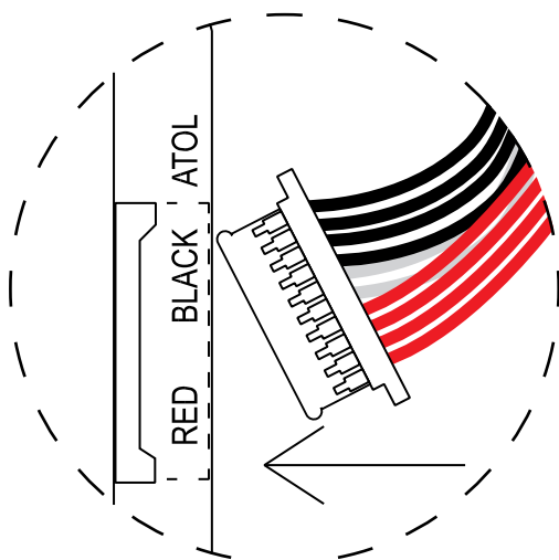
Рисунок 11. Указание цветов
