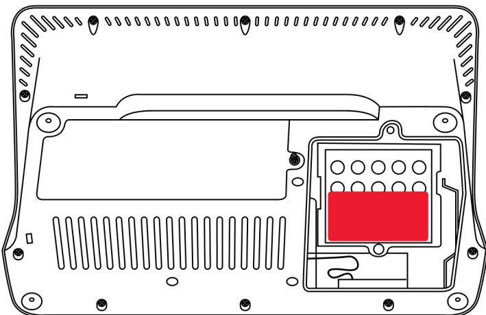
Рисунок 9. Установленный аккумулятор
